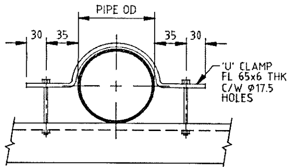
1 'U' CLAMP
