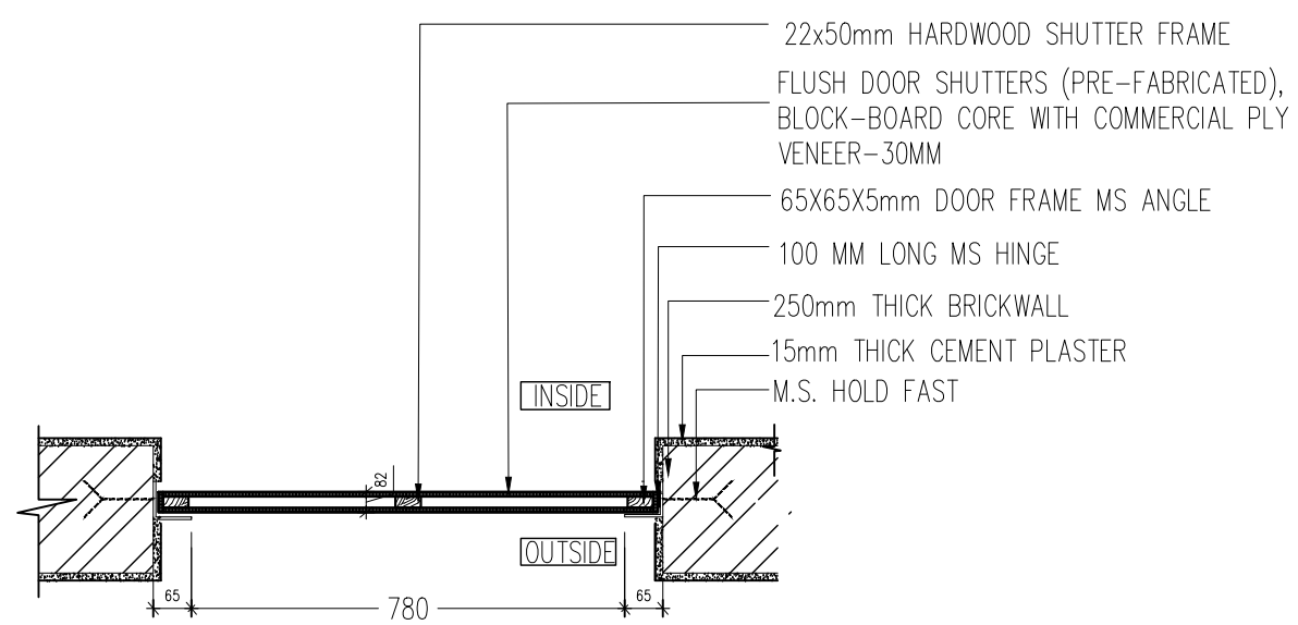
PLAN A-A
