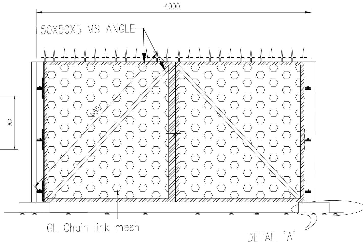
ELEVATION
