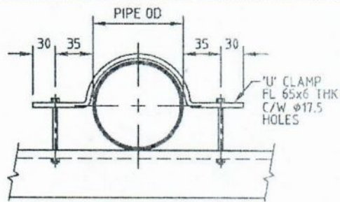
1 'U' CLAMP
