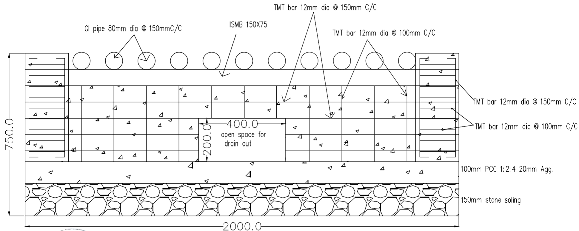
Section A-A
